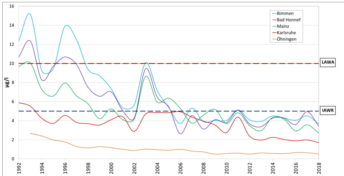
Abbildung 2: Darstellung der EDTA-Konzentration in \mu\text{g/l} (Jahresmittelwerte) in unfiltrierten Wasserproben der Rheinmessstellen von 1992 bis 2018. Der Zielwert der IAWR ( 5 \mu\text{g/l} ) und die LAWA-Zielvorgabe ( 10 \mu\text{g/l} ) sind durch horizontale Linien markiert. An der Messstelle Öhningen wurde EDTA erst ab 1993 im Rhein gemessen.
