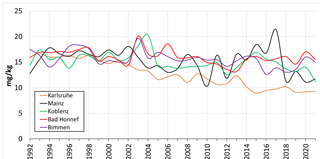
Abbildung 1: Jahresmittelwerte der Arsenkonzentration [mg/kg] in Schwebstoffen im Rhein von 1992 bis 2021. Für die Jahre 1992 und 1994 liegen keine Daten für die Messstelle Karlsruhe vor.
