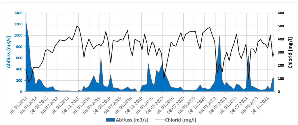
Abbildung 2: Darstellung der Chloridkonzentrationen (Einzelproben) in mg/l als Linie (schwarze Achse) und des täglichen Abflusses (Bezugspegel Perl) in m 3 /s als Fläche (blaue Achse) an der Mosel, gemessen an der Messstation Palzem von 2018 bis 2021. In den Einzelproben werden wiederkehrende Überschreitungen des Orientierungswertes von 200 mg/l sichtbar.
