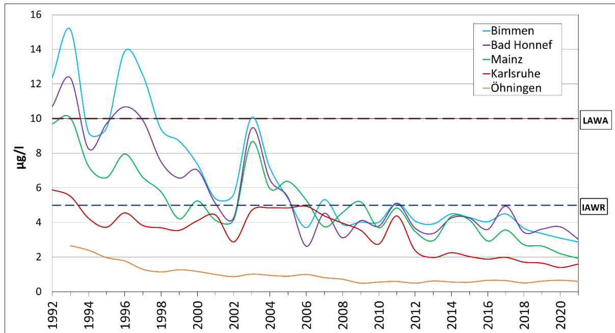
Abbildung 2: Darstellung der EDTA-Konzentration in \mu\text{g/l} (Jahresmittelwerte) in unfiltrierten Wasserproben der Rheinsmessstellen von 1992 bis 2021. Der Zielwert der IAWR ( 5 \mu\text{g/l} ) und die LAWA-Zielvorgabe ( 10 \mu\text{g/l} ) sind durch horizontale Linien markiert. An der Messstelle Öhningen wurde EDTA erst ab 1993 gemessen.
