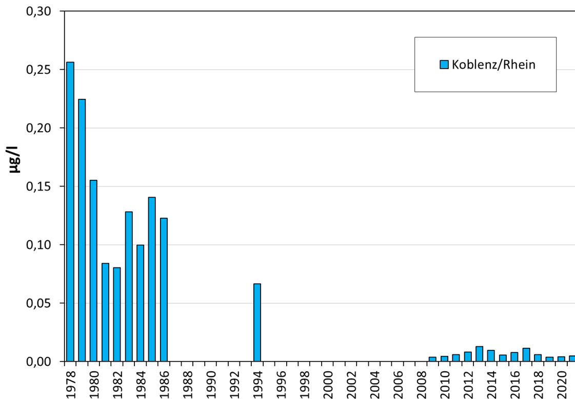
Abbildung 2: Zeitlicher Verlauf der Quecksilberkonzentration (Jahresmittelwerte) in Wasserproben (unfiltriert), beispielhaft an der Messstelle Koblenz/Rhein von 1978 bis 2021. In den Jahren 1987 bis 1993 und 1995 bis 2008 lagen die Jahresmittel unterhalb der Bestimmungsgrenze und wurden in dieser Grafik nicht dargestellt. Ab 2009 sind durch die Verwendung einer Methode mit niedriger Bestimmungsgrenze wieder Messwerte verfügbar.
